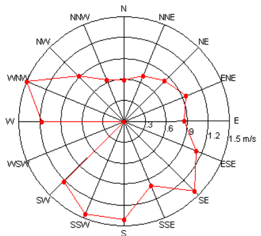
Velocitat del vent - Unitat Mòbil 3 - 10/04/2025 al 09/06/2025
