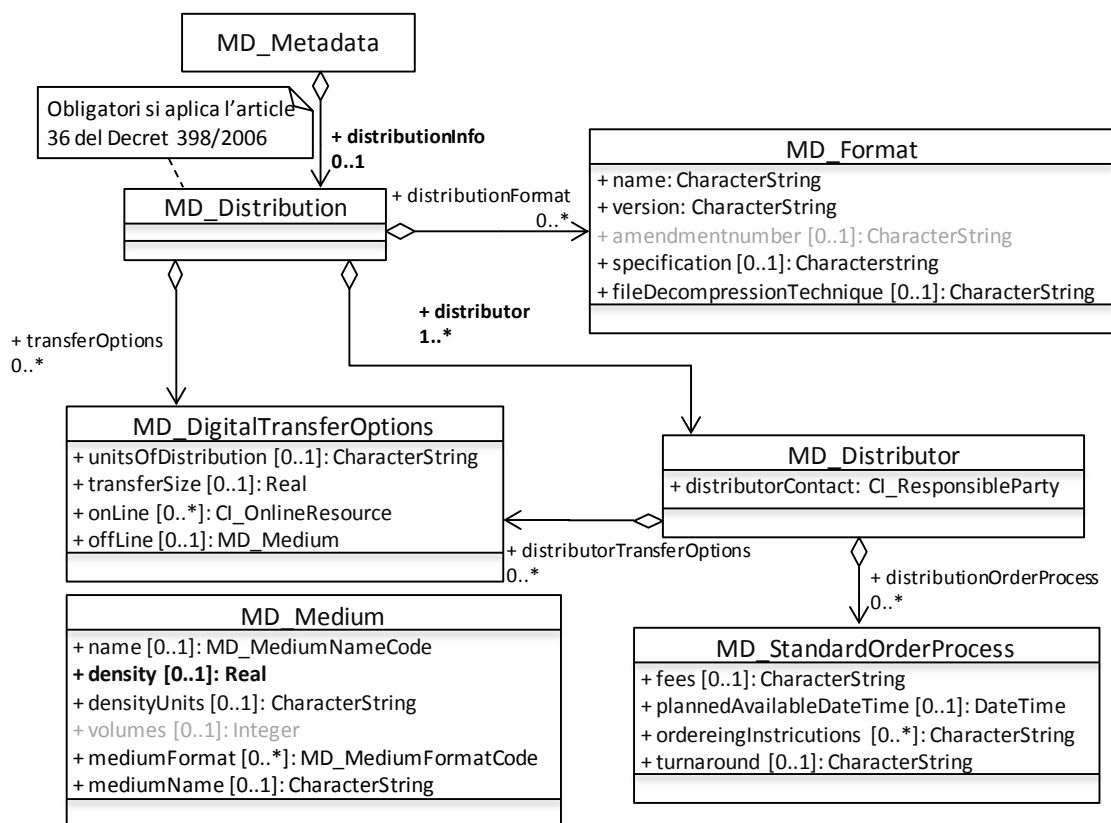
Figura 9 Esquema UML segons ISO19115
