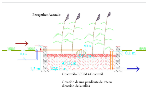
Plànol sistema de depuració C.I. Fogars. Font: Arxiu PNM
