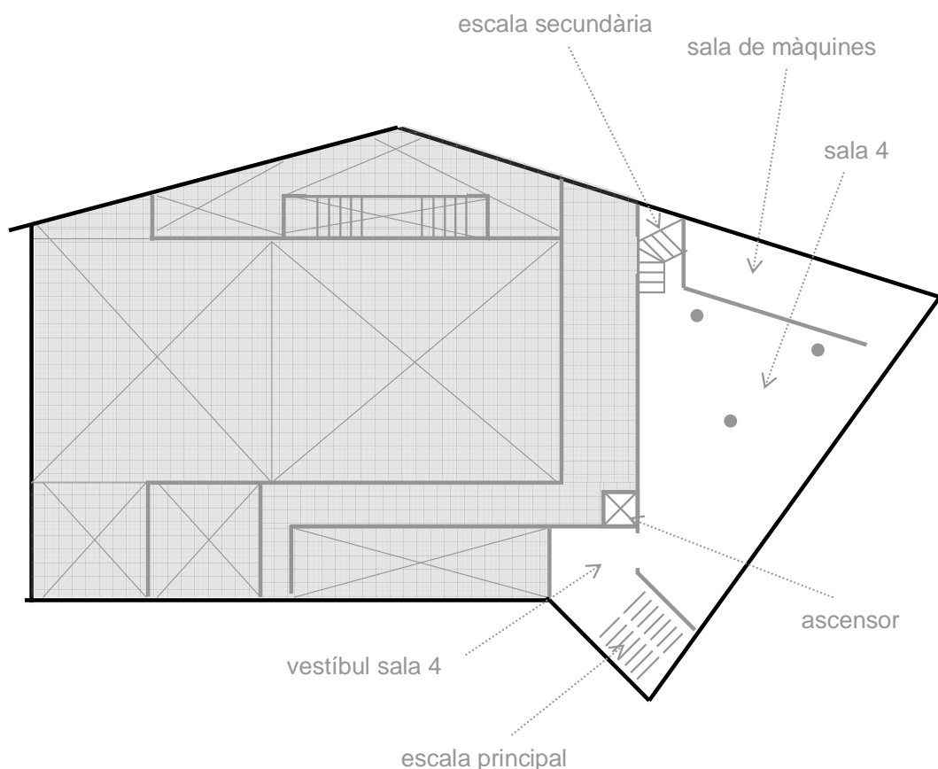
Planta 2 179m 2
