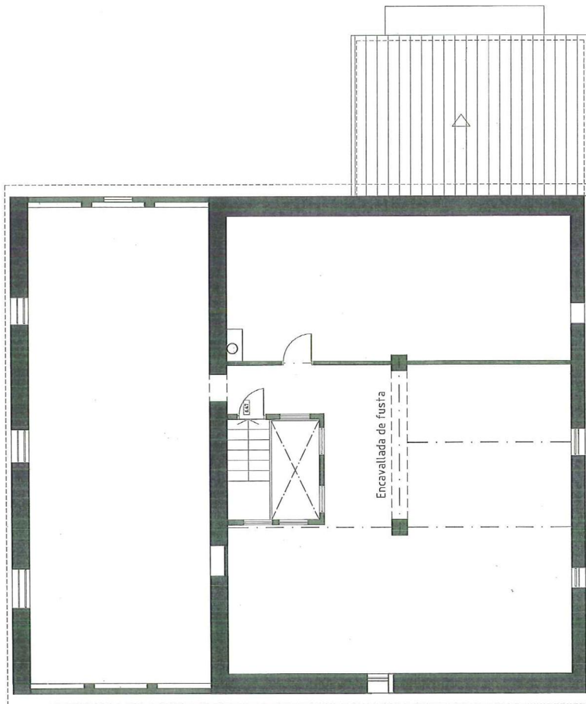
PLANTA SOTACOBERT
